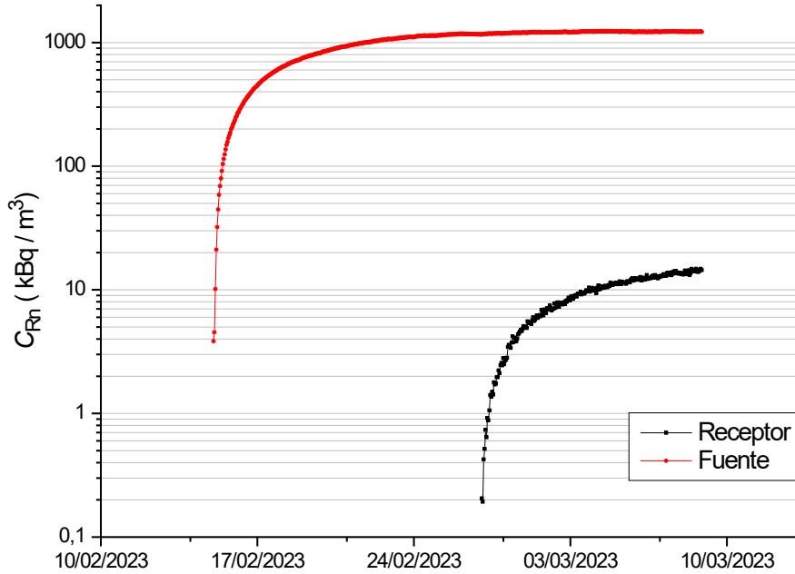
Fig. 1. Evolución de la concentración de radón en la cámara primaria/fuente (rojo) y en la cámara secundaria/receptor (negro) durante el ensayo. Radon concentration evolution in the primary/source chamber (red) and in the secondary/receiver container (black) during the test.
